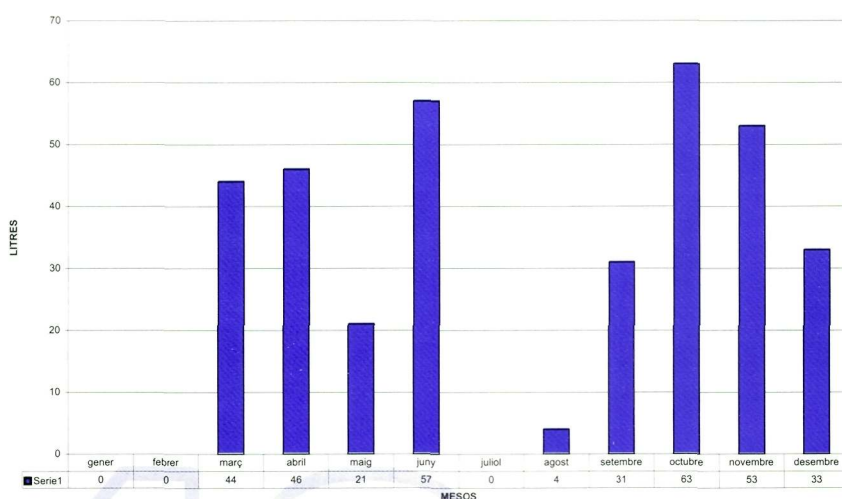
PLUVIOMETRIA D'ALPICAT ANY 2000. (total l/m 2 :352)
